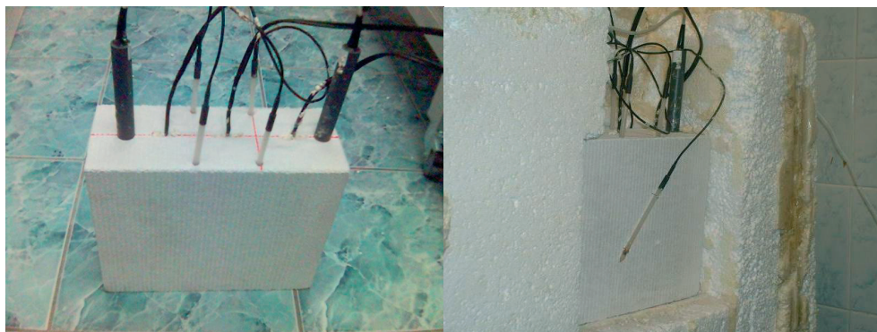
Rys. 2. Próbką betonu komórkowego 600 zastosowana do badania współczynnika przewodzenia ciepła.
