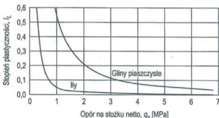
Rys. 5. Nomogram zależności I_L od q_c wg Młynarka [11]
