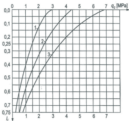
Rys. 4. Nomogram zależności I_L od q_c wg Wiłuna [10]
