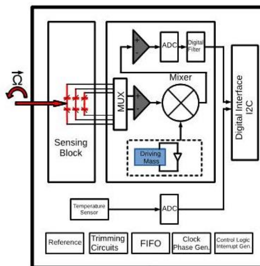
Rys. 2. Schemat funkcjonalny elektronicznego żyroskopu L3GD20 [10]
