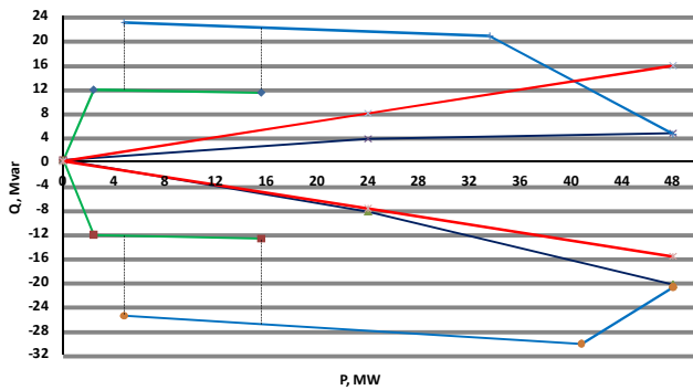
Rys. 7. Obszar możliwej generacji mocy biernej przez przykładową farmę wiatrową o mocy 48 MW (na poziomie 110 kV) dla różnych wartości mocy czynnej wiatraków farmy, przy pracy w obszarze dopuszczalnych wartości współczynnika mocy wraz z uwzględnieniem regulacji specjalnej
