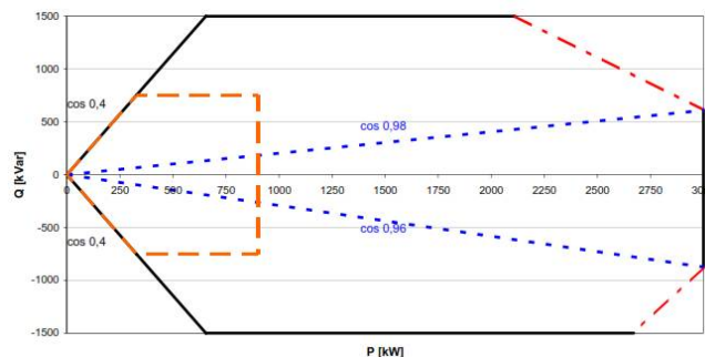
Rys. 6. Dopuszczalny obszar pracy pojedynczego wiatraka Vestas V90 3 MW przy różnych wartościach generowanej (pobieranej) mocy biernej z uwzględnieniem regulacji specjalnej [3]
