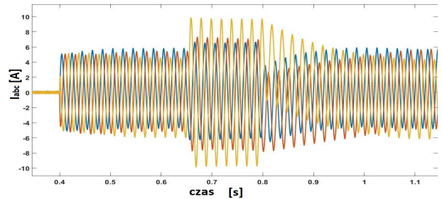
Rys. 6. Przebieg prądu na wyjściu pierwszego przekształtnika podczas powstania krótkotrwałej przerwy w fazie L1 przekształtnika 2
