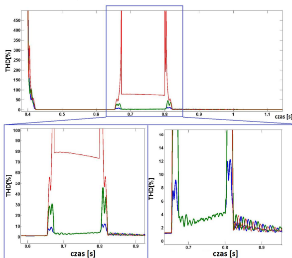
Rys. 10. THD prądu na trzech fazach, na wyjściu jednocanałowego przekształtnika w trakcie trwania zakłócenia typu przerwa w fazie. W czasie 0,1–0,4 s przekształtnik nie oddaje energii do sieci
