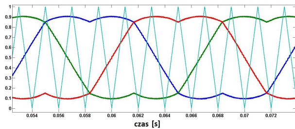
Rys. 2. Sygnał modulujący i modulowany w układzie sterowania VOC
