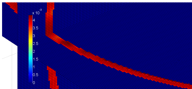
Rys. 5. Rozkład pola elektrycznego w skórze pokrywającej kulę tuszczu znajdującej się w polu magnetycznym, wynik po zastosowaniu filtra dolnoprzepustowego
