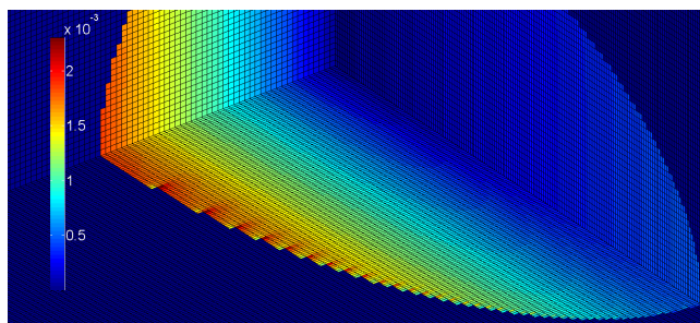
Rys. 1. Rozkład pola elektrycznego w elipsoidzie znajdującej się w polu magnetycznym, wynik bezpośrednio ze środowiska symulacyjnego
