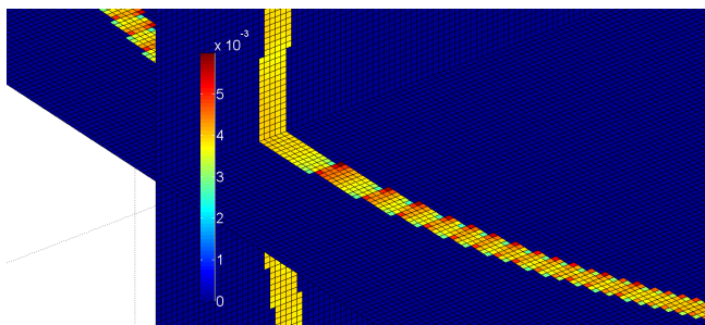
Rys. 2. Rozkład pola elektrycznego w skórze pokrywającej kulę tłuszczu znajdującej się w polu magnetycznym, wynik bezpośrednio ze środowiska symulacyjnego
