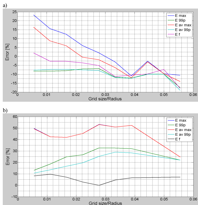
Rys. 6. Błąd wartości maksymalnej pola elektrycznego w zależności od stosunku rozdzielczości siatki do promienia kuli/dłuższej półosi elipsoidy dla różnych wielkości opisujących poziom ekspozycji ( E_{max} – błąd bezpośrednio z symulacji, E_{99p} – błąd przyjmując jako wartość maksymalną wartość 99 centyla z wyników bezpośrednio z symulacji, E_{av\ max} – błąd po uśrednieniu wektorowym zgodnym z ICNIRP, E_{av\ 99p} – błąd przyjmując jako wartość maksymalną wartość 99 centyla z wyników po uśrednieniu ICNIRP, E_f – błąd po zastosowaniu filtra dolnoprzepustowego), a) wyniki dla elipsoidy, b) wyniki dla kuli tuszczu pokrytej warstwą skóry
