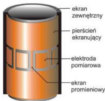
Rys. 2. Schemat jednopłaszczyznowego czujnika ECT
