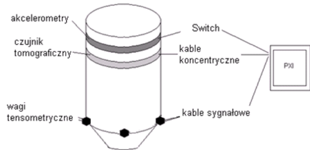
Rys. 5. Schemat rozmieszczenia urządzeń pomiarowych i sensorów na zbiorniku transportowym
