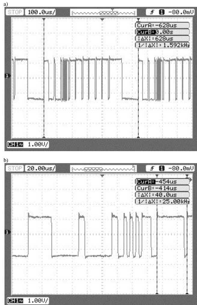
Rys. 4. Oscylogramy DMX512: a) Cały pakiet w przypadku sterowania 8 kanałów, b) początek pakietu dla wartości pierwszych trzech pakietów 0 (00000000b), 170 (10101010b) i 255 (11111111b)
