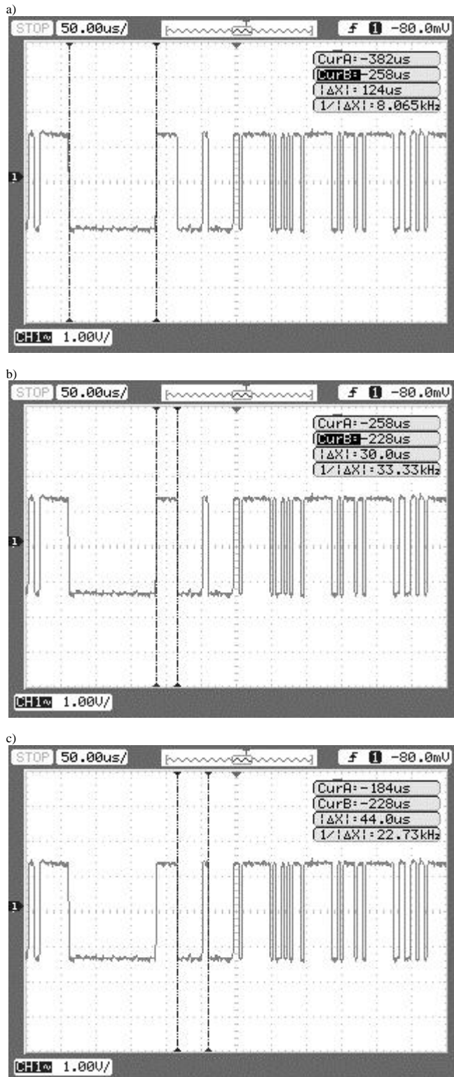
Rys. 3. Oscylogramy DMX512: a) sygnał Break, b) MAB – Mark after Break, c) pierwszy slot
