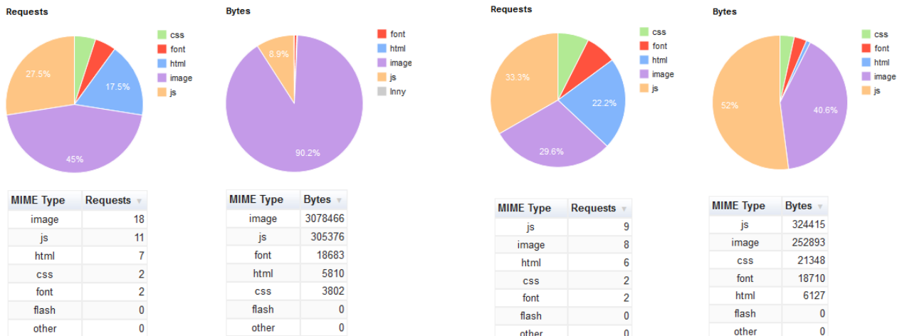
Rys. 11. Analiza elementów strony przed optymalizacją wg WebPageTest
