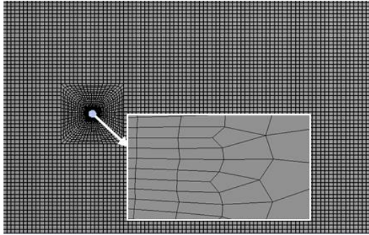
Rys. 6. Siatka obliczeniowa
