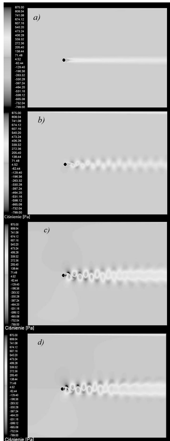
Rys. 7. Rozkład ciśnienia całkowitego dla: a) 7 395 elementów, b) 57 735 elementów, c) 393 360 elementów, d) 611 400 elementów
