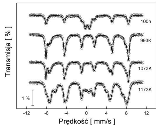
Rys. 5. Widma mössbauerowskie ceramicznych próbek (\text{BiFeO}_3)_{0.9}\text{-(BaTiO}_3)_{0.1} otrzymanych w procesie aktywacji mechanicznej po 100 h oraz poddanej obróbce termicznej w różnych temperaturach
