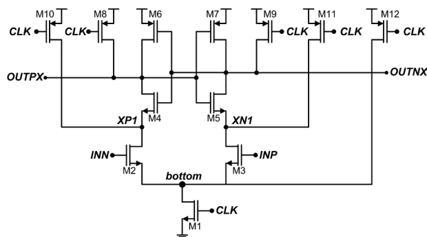
Rys. 4. Schemat synchronicznego zatrasku
