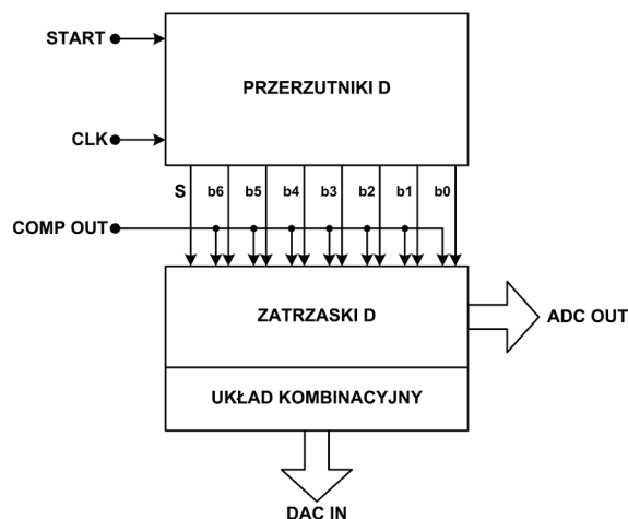
Rys. 5. Schemat pojedynczej komórki rejestru kolejnych przybliżeń
