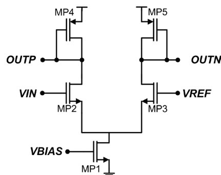
Rys. 3. Schemat przedwzmacniacza
