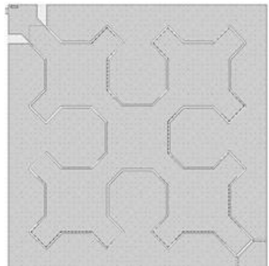
Fig. 6. Layout of Sierpiński MIM 2
