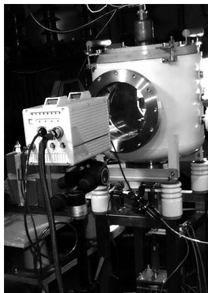
Rys. 2. Rejestracja zdjęć przy użyciu ultra-szybką kamery
