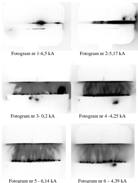
Rys. 6. Fotografy zarejestrowane podczas prób łączeniowych prądu 6,14 kA dla styków wyposażonych nakładki z nacięciami promieniowymi
