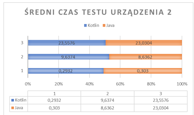
Rys. 2. Średni czas wykonania testów na NR2.
