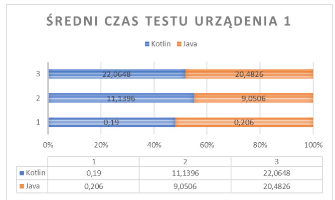
Rys. 1. Średni czas wykonania testów na NR1.
