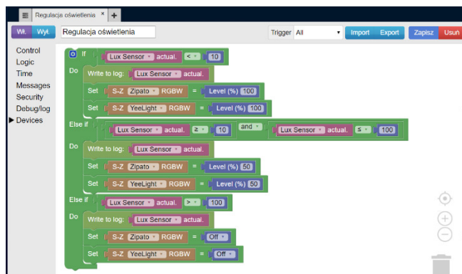
Rys. 5. Skrypt wydarzenia „Regulacja oświetlenia”
